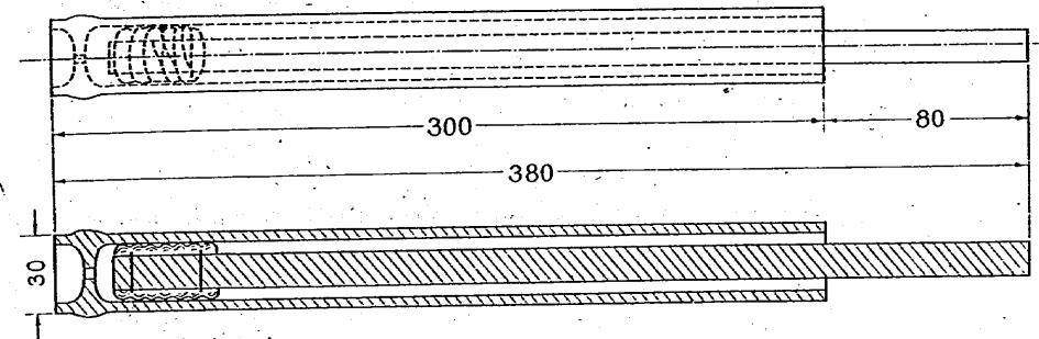
押シ出シ棒ノツクリ方
